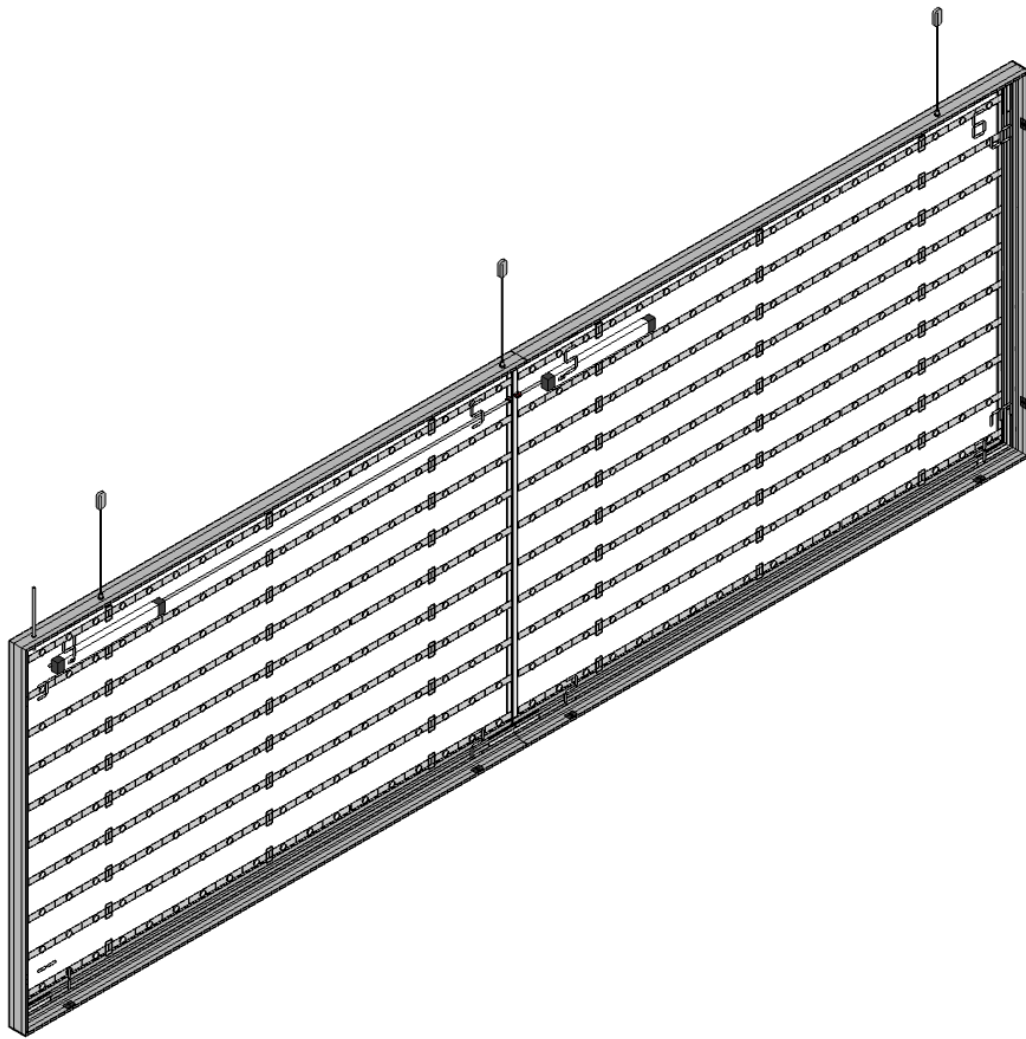
Tył ramy
