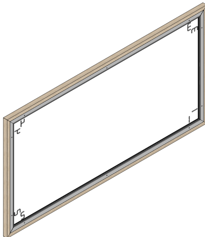
Tył ramy
